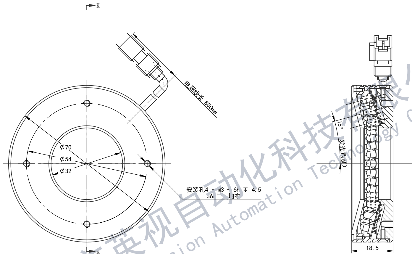
剖面 K-K
